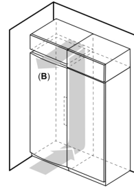
B: Sortie d'air \geq 200 \text{ cm}^2
