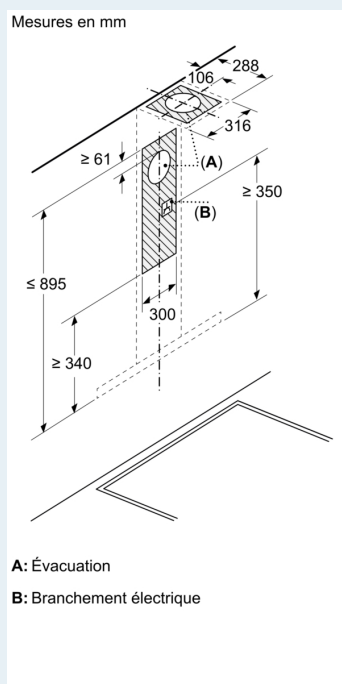
Mesures en mm Appareil en mode d'évacuation d'air
