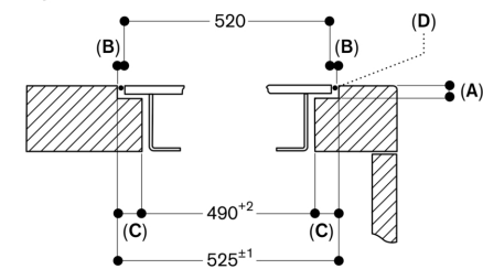
A: 6,5 +0,5 B: 2,5 C: 17,5 D: Remplissage avec du silicone Mesures en mm
