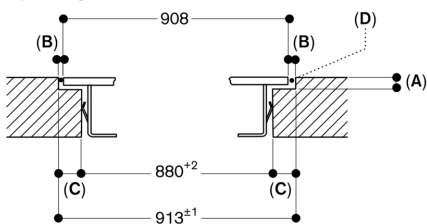
A: 6,5 +0,5 B: 2,5 C: 16,5 D: Remplissage avec du silicone Mesures en mm
