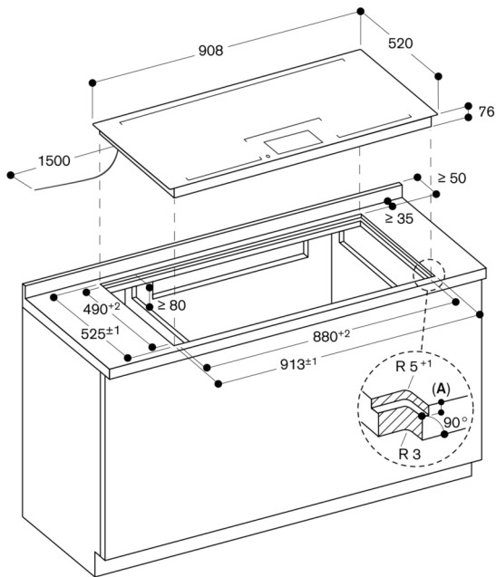
A: 6,5 +0,5 Mesures en mm
