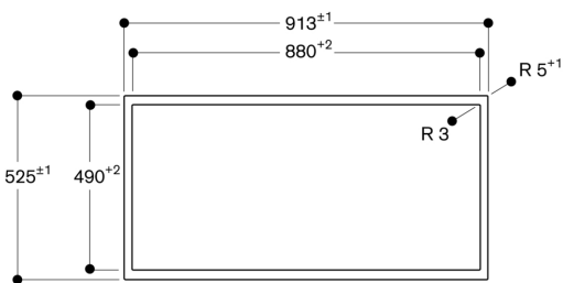
Mesures en mm
