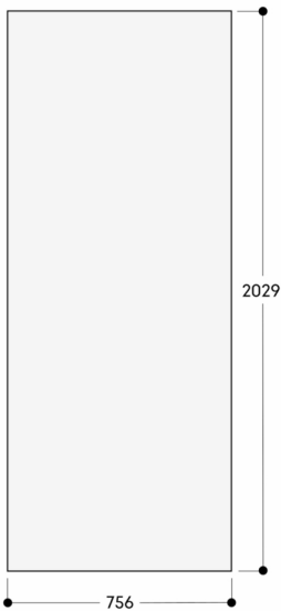
Le panneau d'habillage fait 19 mm d'épaisseur Les dimensions maximales des panneaux d'habillage sont basées sur un jeu de 3 mm, sur la base d'une seule niche Mesures en mm
