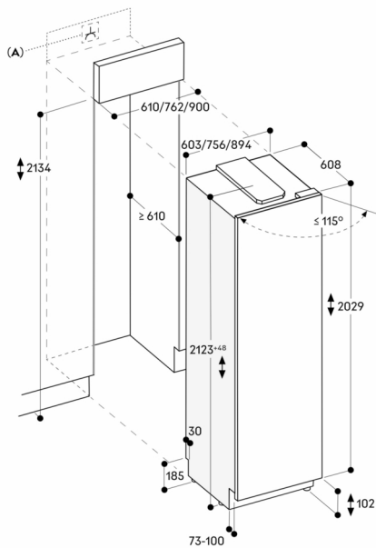
A: Branchement électrique Les dimensions maximales du panneau de porte sont basées sur un dégagement de 3 mm La hauteur de la plinthe peut être réduite à 50 mm Mesures en mm
