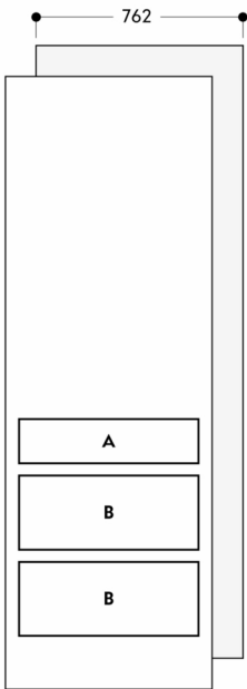
A: Tiroir fraîcheur B: Tiroir fraîcheur avec contrôle de température et d'humidité Mesures en mm
