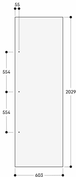
Le panneau d'habillage fait 19 mm d'épaisseur Les dimensions maximales des panneaux d'habillage sont basées sur un jeu de 3 mm, sur la base d'une seule niche Mesures en mm
