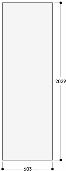
Le panneau d'habillage fait 19 mm d'épaisseur Les dimensions maximales des panneaux d'habillage sont basées sur un jeu de 3 mm, sur la base d'une seule niche Mesures en mm
