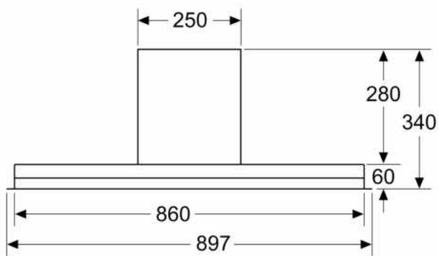
mesures en mm Vue de face
